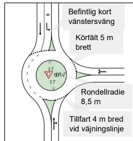
Figur 21. Schematisk skiss över cirkulationsplats, dimensioner enligt Göteborg Stads Tekniska handbok
