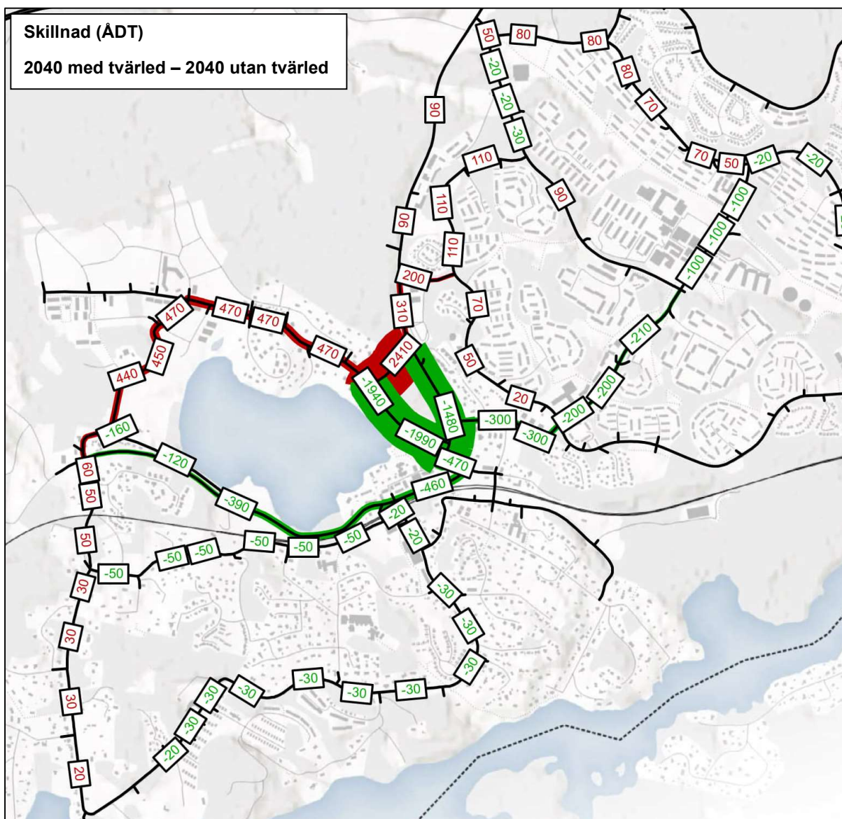
Figur 13. Effekt på trafiken i framtiden med tvärled Södra Hallsta utbyggd (skillnad i ÅDT).
