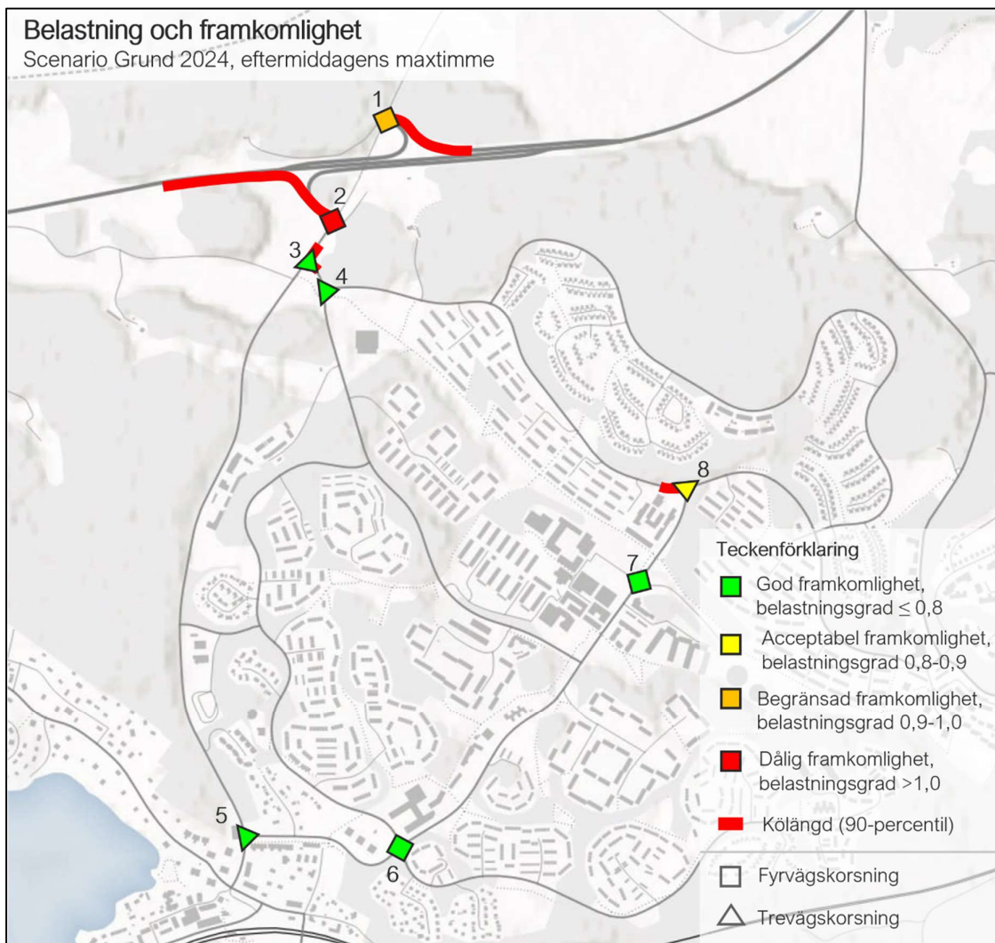
Figur 18. Belastning och framkomlighet under eftermiddagens maxtimme i korsning 1–8, framtidsscenario 2040. © Lantmäteriet
