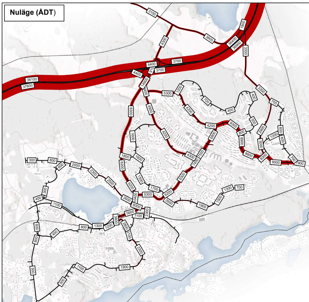
Figur 10. Beräkning av trafik i nuläget (ÅDT), för kalibrering av modell.
