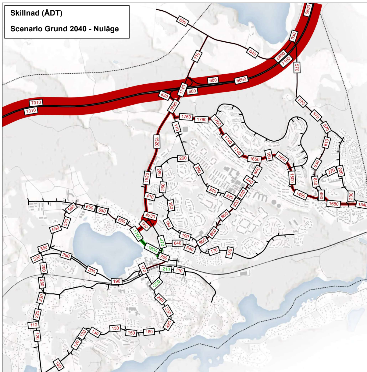
Figur 12. Ökning av trafiken i det prognosstyrda framtidsscenarioet år 2040 jämfört med nuläget (skillnad i ÅDT).
