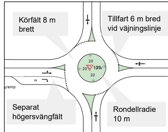
Figur 20. Schematisk skiss över cirkulationsplats med ett separat högersvängfält
