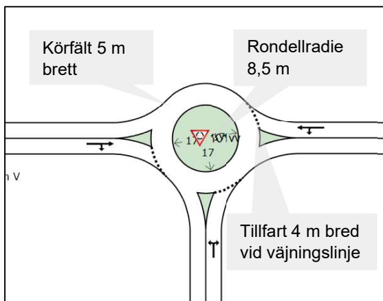
Figur 22. Schematisk skiss över cirkulationsplats, dimensioner enligt Göteborg Stads Tekniska handbok.
