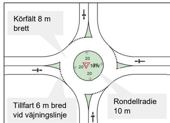
Figur 19. Schematisk skiss över cirkulationsplats
