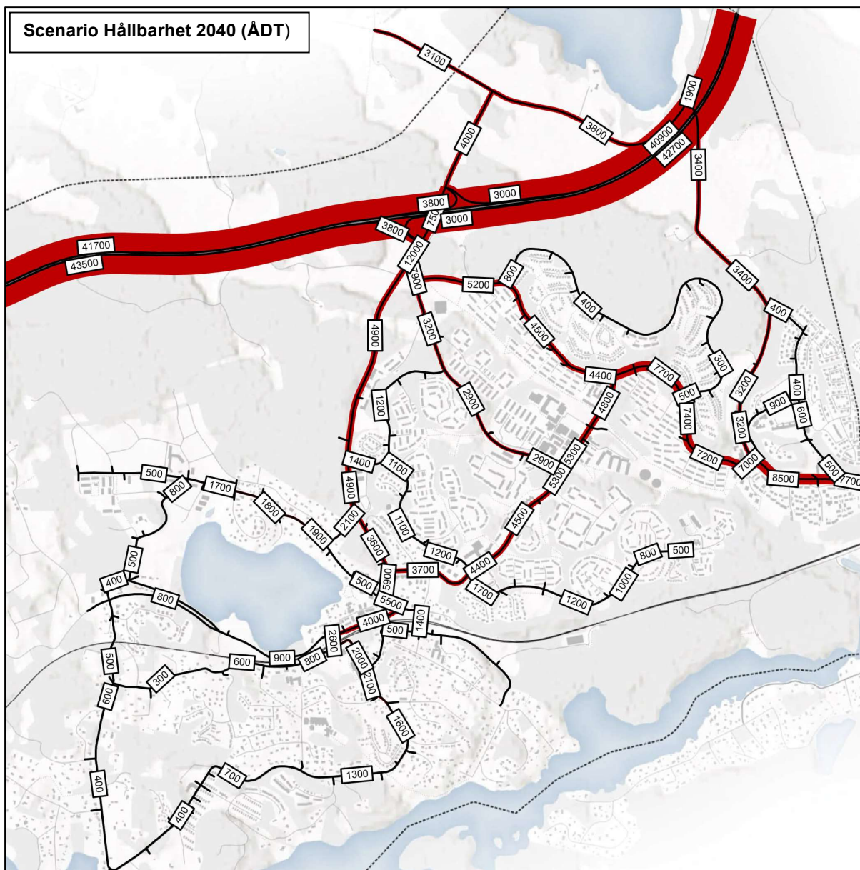
Figur 14. Trafikprognos år 2040 för viljestyrt framtidsscenario Scenario Hållbarhet 2040 (ÅDT).
