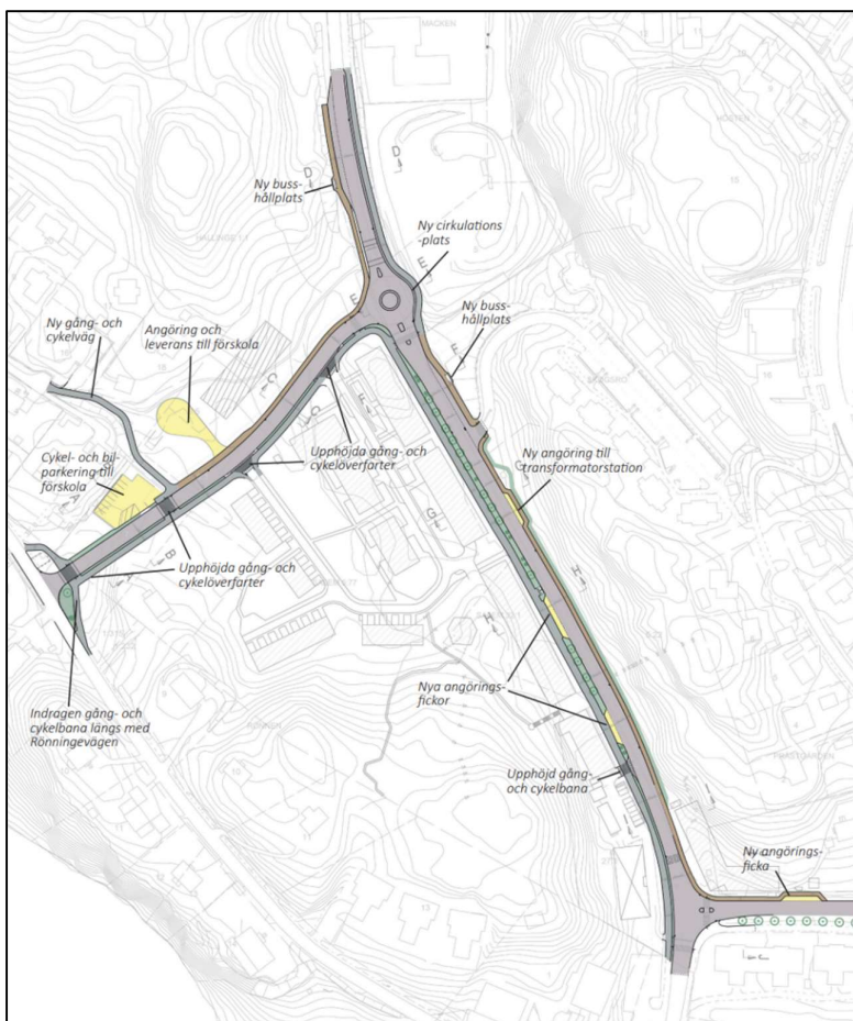
Figur 5. Skiss på planerad ny tvärled Södra Hallsta.
